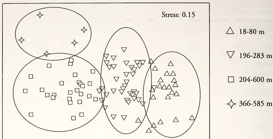
Figure 2. Multidimensional scaling ordination analysis for the five surveys. Figura 2. Análisis de ordenación de escalamiento multidimensional para las cinco campañas.
